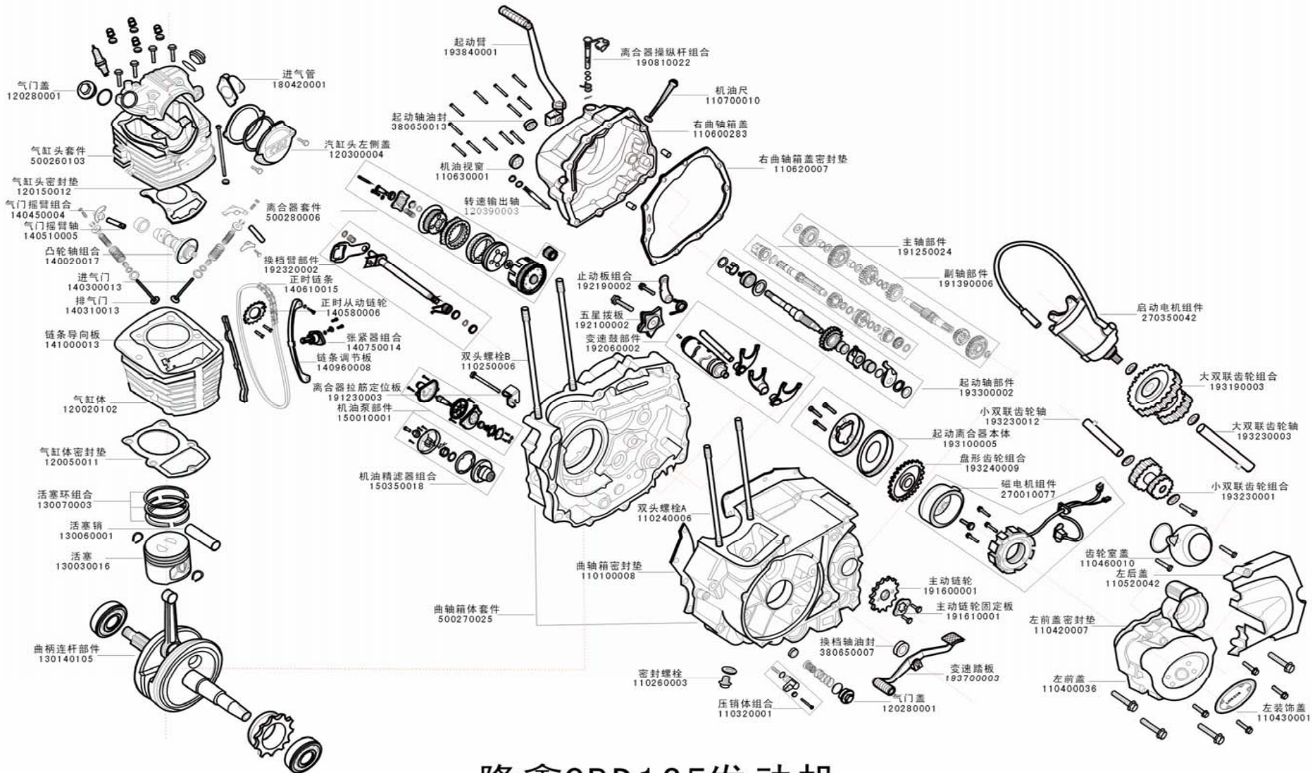
隆鑫CBD125发动机
